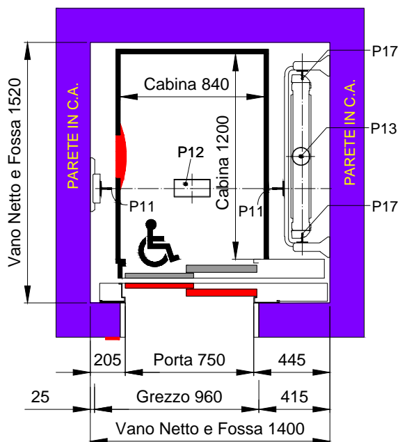
PIANTA VANO CORSA
